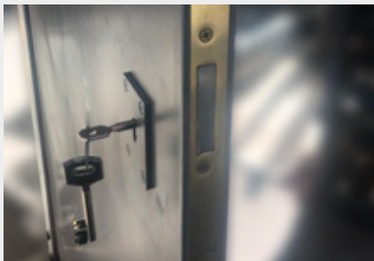
01. Cerradura de tres puntos, uno central con llave de gorja y un anclaje inferior y superior contra el marco
